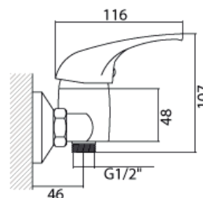
Planos Técnicos
